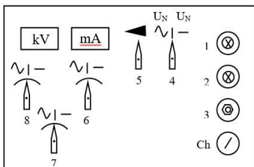
Fig. 2 – Pupitrul de comandă al sursei WPT 4,4/100.
